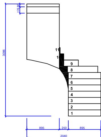
ČELNÍ POHLED
