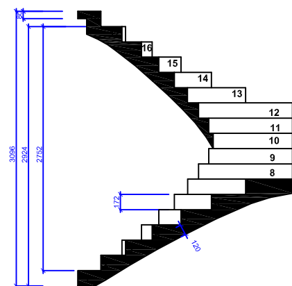
BOČNÍ POHLED
