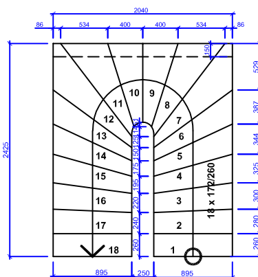
PŮDORYS
