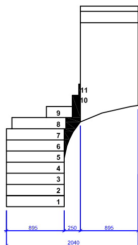
BOČNÍ POHLED
