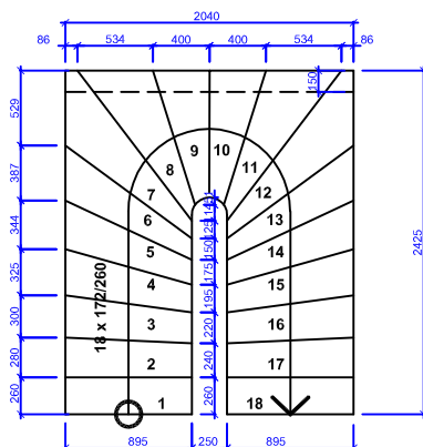
PŮDORYS
